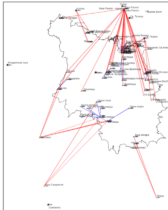
СХЕМА GPS мрежата
